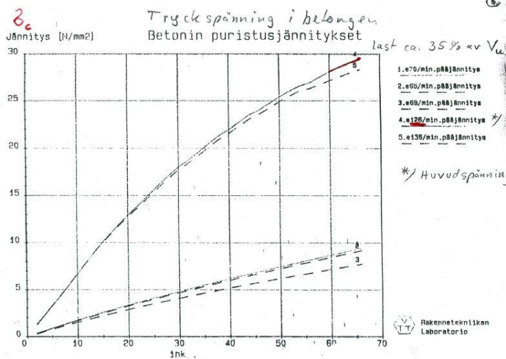
Kuva 2. FEM analyysillä ja epälineaarilla materiaalimallilla laskettu pääjämnityksen taso laatan alapinnassa (elementti 126). Vastaavan rakenteen lävistyskoe TTKK:lla.
